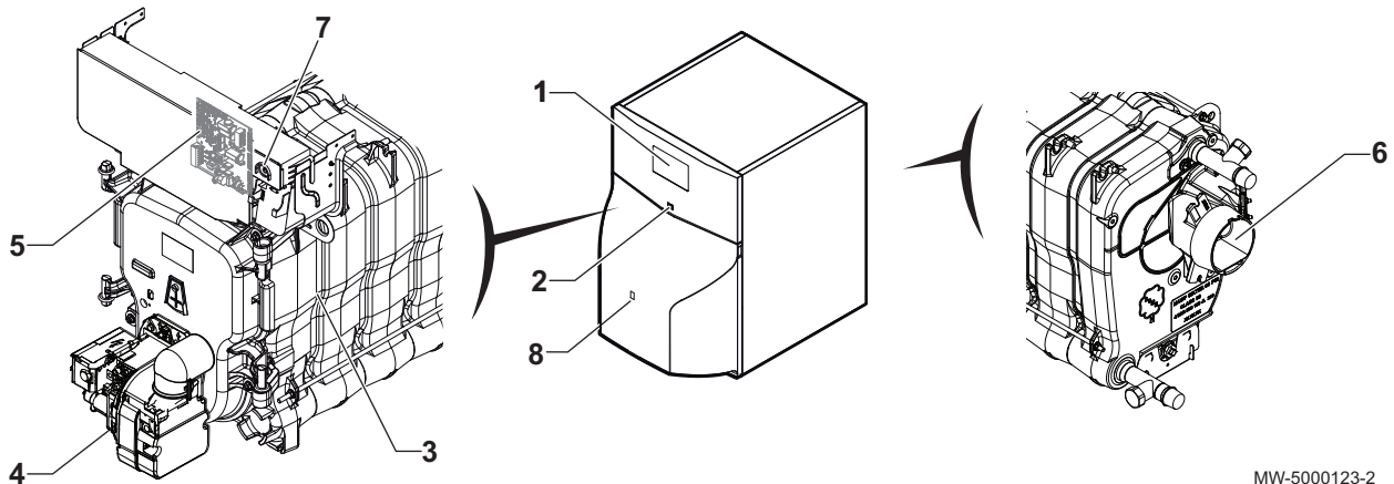
Abb.2 Hauptkomponenten
