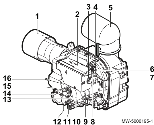
Abb.3 Hauptkomponenten
